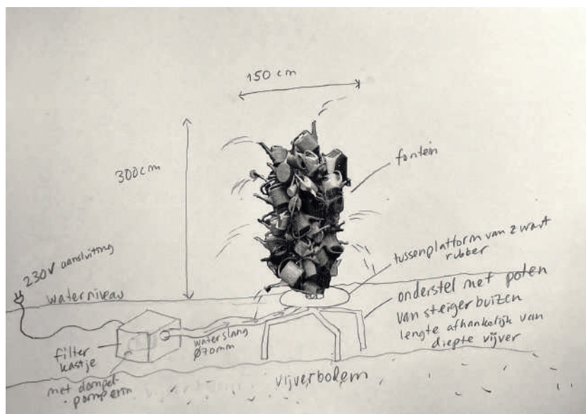
Technische tekening, mogelijkheid 2.
